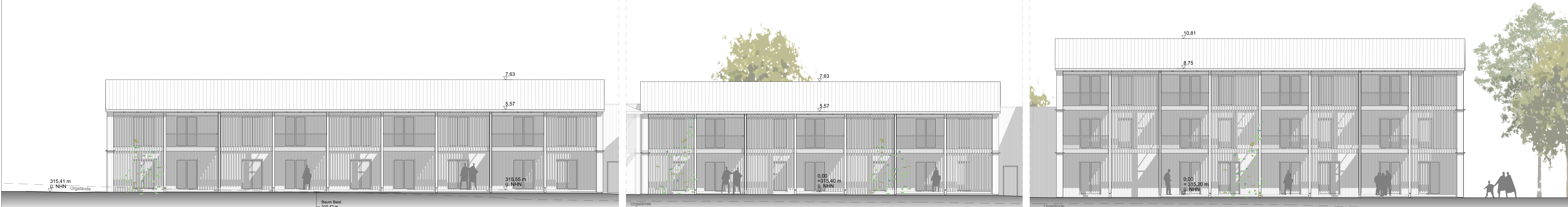
Ansicht Nord-Ost
