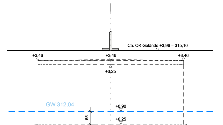
Ansicht West
