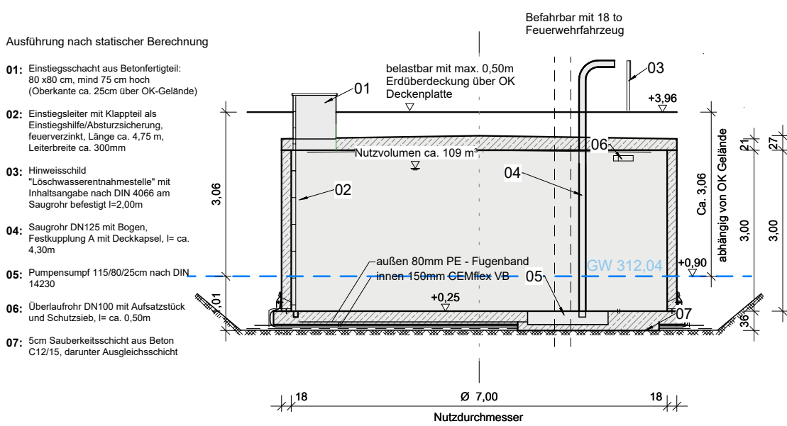
Schnitt A-A
