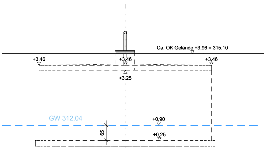
Ansicht Ost
