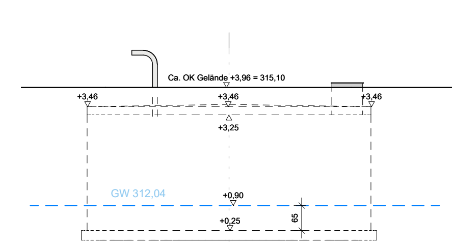
Ansicht Süd
