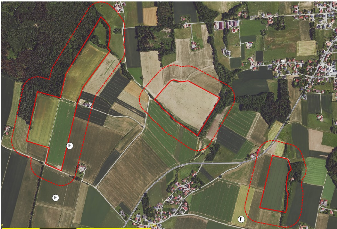
Abbildung 12: Lage der Revierzentren der Feldlerche (F); rot durchgezogen: Grenzen der geplanten Solarparks, rot gestrichelte Linie: 100-Meter-Puffer. Hintergrund Quelle: https://geoportal.bayern.de/bayernatlas/ )
